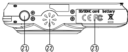
底部視圖
